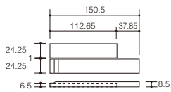
ECP-2515NB タイル形状図(詳細)
