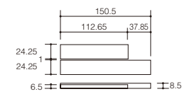
ECP-2515TNA タイル形状図(詳細)
