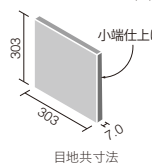
ECP-3031T/*(R)
