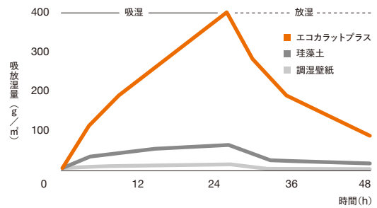
各壁材の吸放湿量
