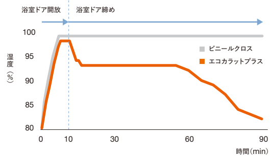
脱衣所での湿度調整効果
