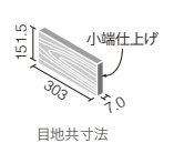
ECP-3151T/**(R)
