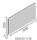
ECP-630
