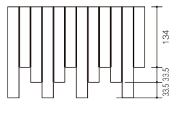
ECP-2520TN シート形状図(詳細)
