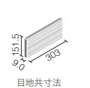
ECP-315/**AN
