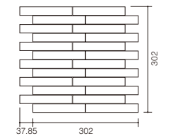
ECP-2515NET シート形状図(詳細)
